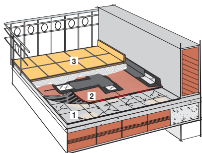
1 Vecchia pavimentazione. 2 SELFTENE TERRACE SYSTEM. 3 Nuova pavimentazione.
